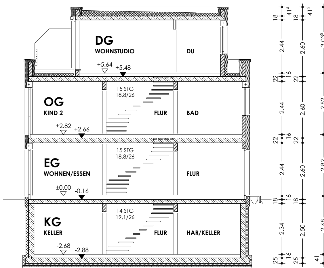
SCHNITT
