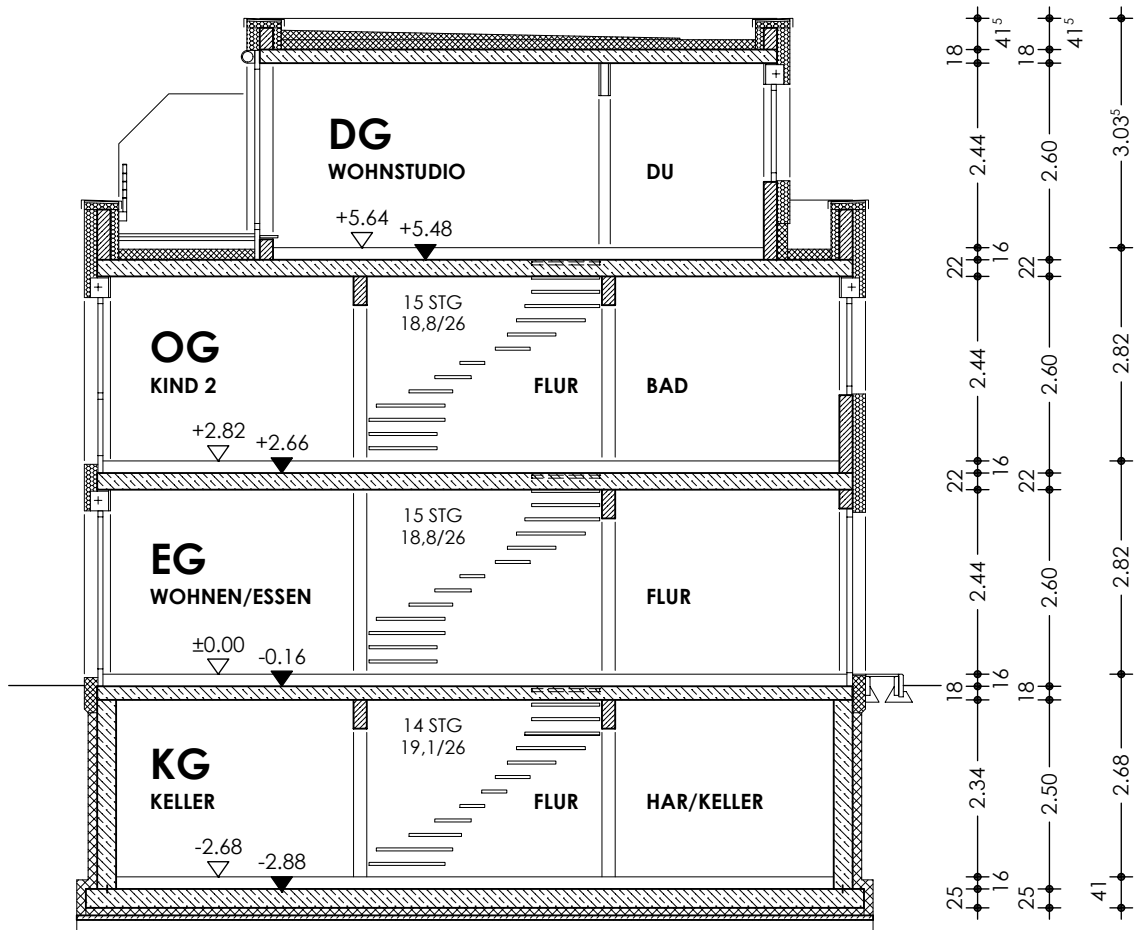
SCHNITT
