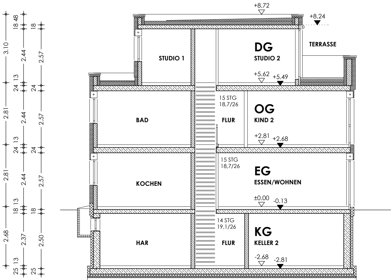
SCHNITT A-A
